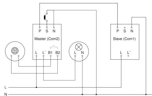
aansluitschema Master/slave koppelin
